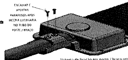
Sistema de fixação em poste / braço reto
